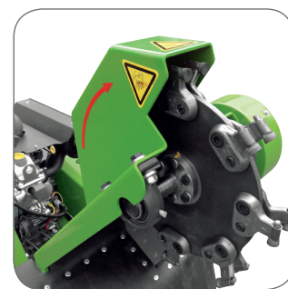
Fräsrads mit 16 Zähnen - werkzeuglos 3-Fach wendbar
